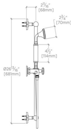
SIDE VIEW SCALE: 1"=1'-0"
