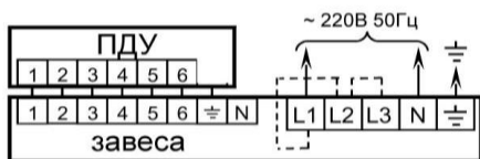
Рис. 3. Схемы подключения занавес к электросети и пульту управления
