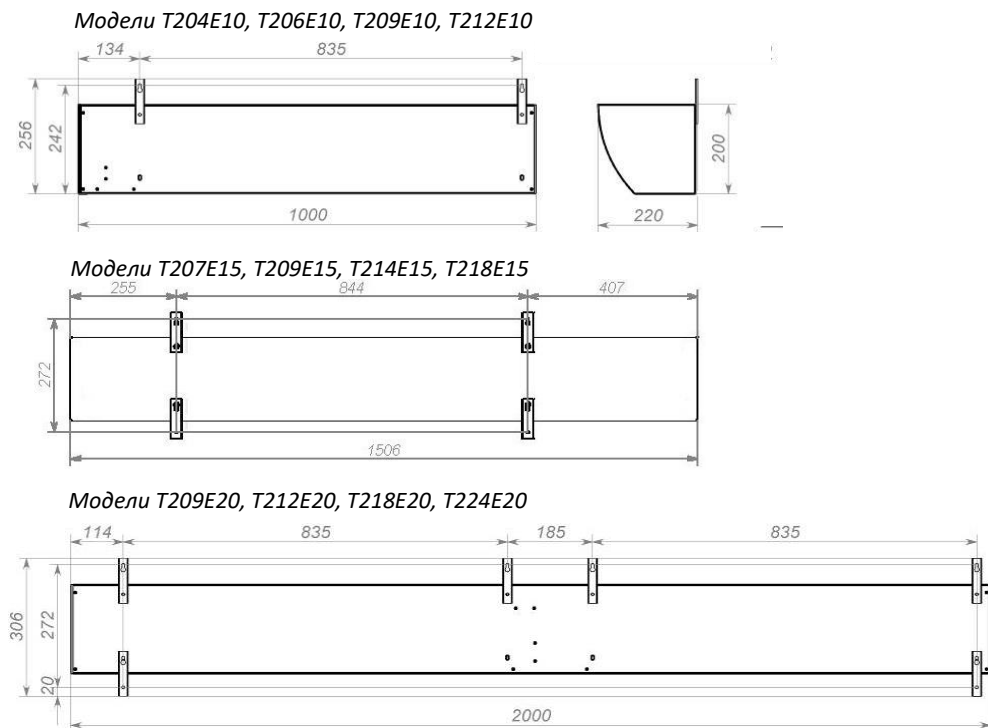
Рис. 2. Габаритные и установочные размеры приборов
