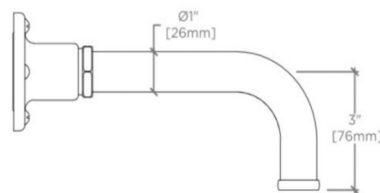
SIDE VIEW SCALE: 3"=1'-0"
