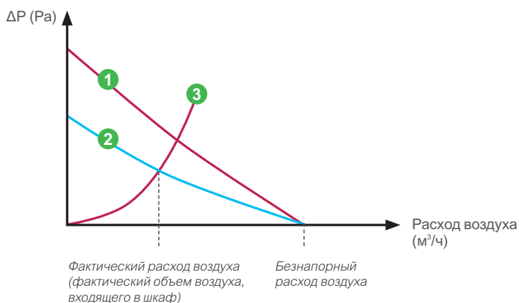
Центробежный вентилятор
