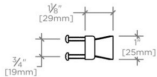
SIDE VIEW SCALE: 3"=1'-0"
