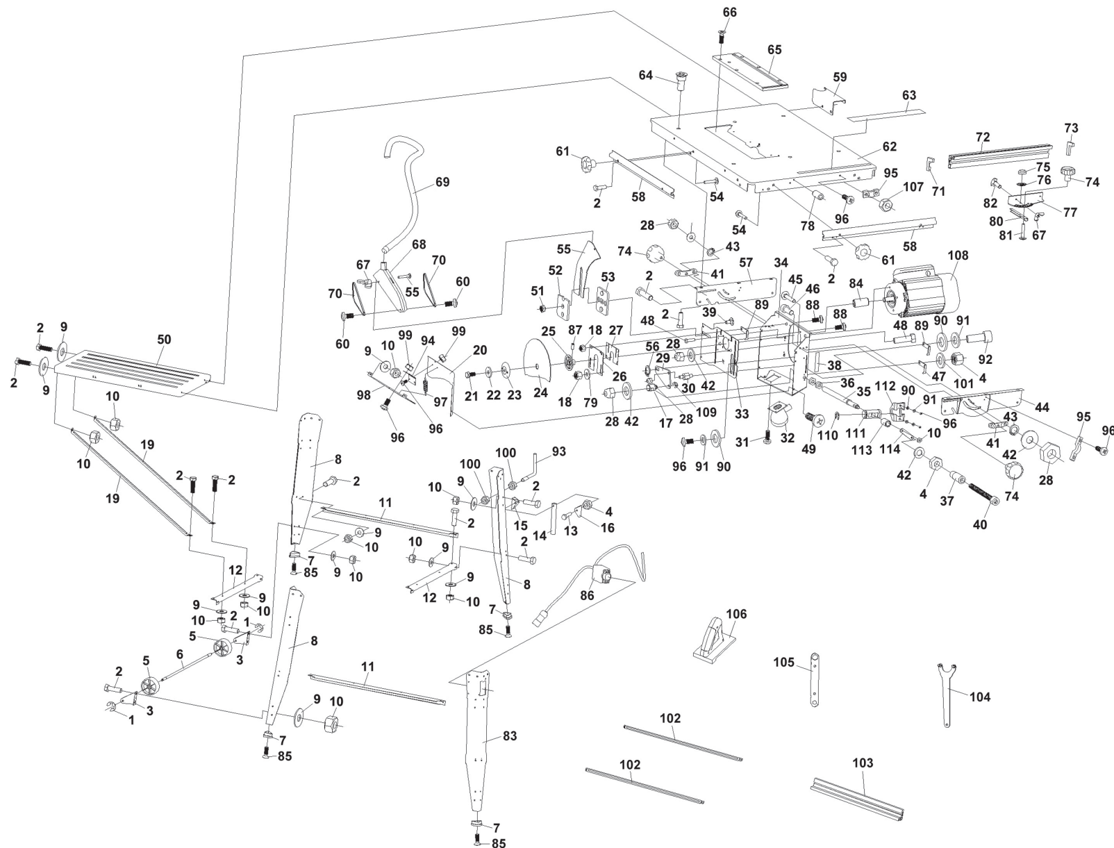
Схема сборки деталей и узлов станка
