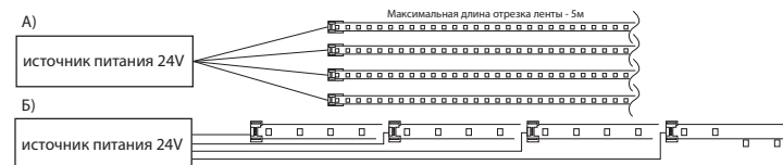
Схема подключения ленты.
