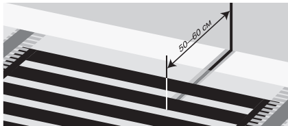
Рис. 5. Расположение датчика температуры пола относительно уложенной пленки
