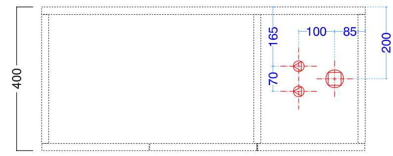
LIGHT30_VERSIONE ISOLA PREDISPOSIZIONE SCARICHI E ADDUZIONE ACQUA
