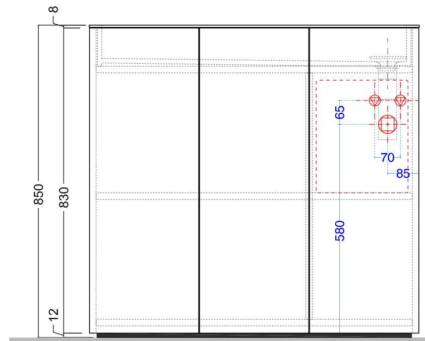
LIGHT30_VERSIONE PARETE PREDISPOSIZIONE SCARICHI E ADDUZIONE ACQUA
