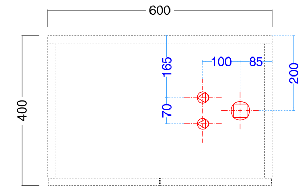
LIGHT30_VERSIONE ISOLA PREDISPOSIZIONE SCARICHI E ADDUZIONE ACQUA
