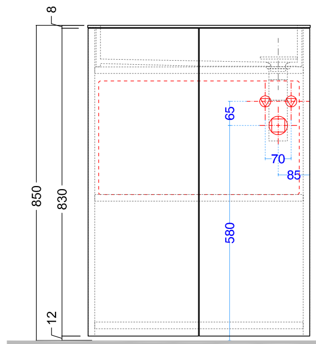
LIGHT30_VERSIONE PARETE PREDISPOSIZIONE SCARICHI E ADDUZIONE ACQUA
