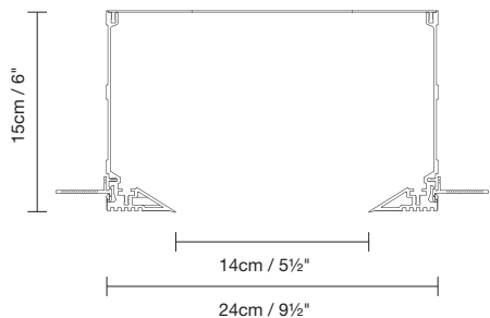
sección caja Deep System
