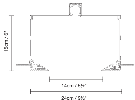
sección caja Deep Track System
