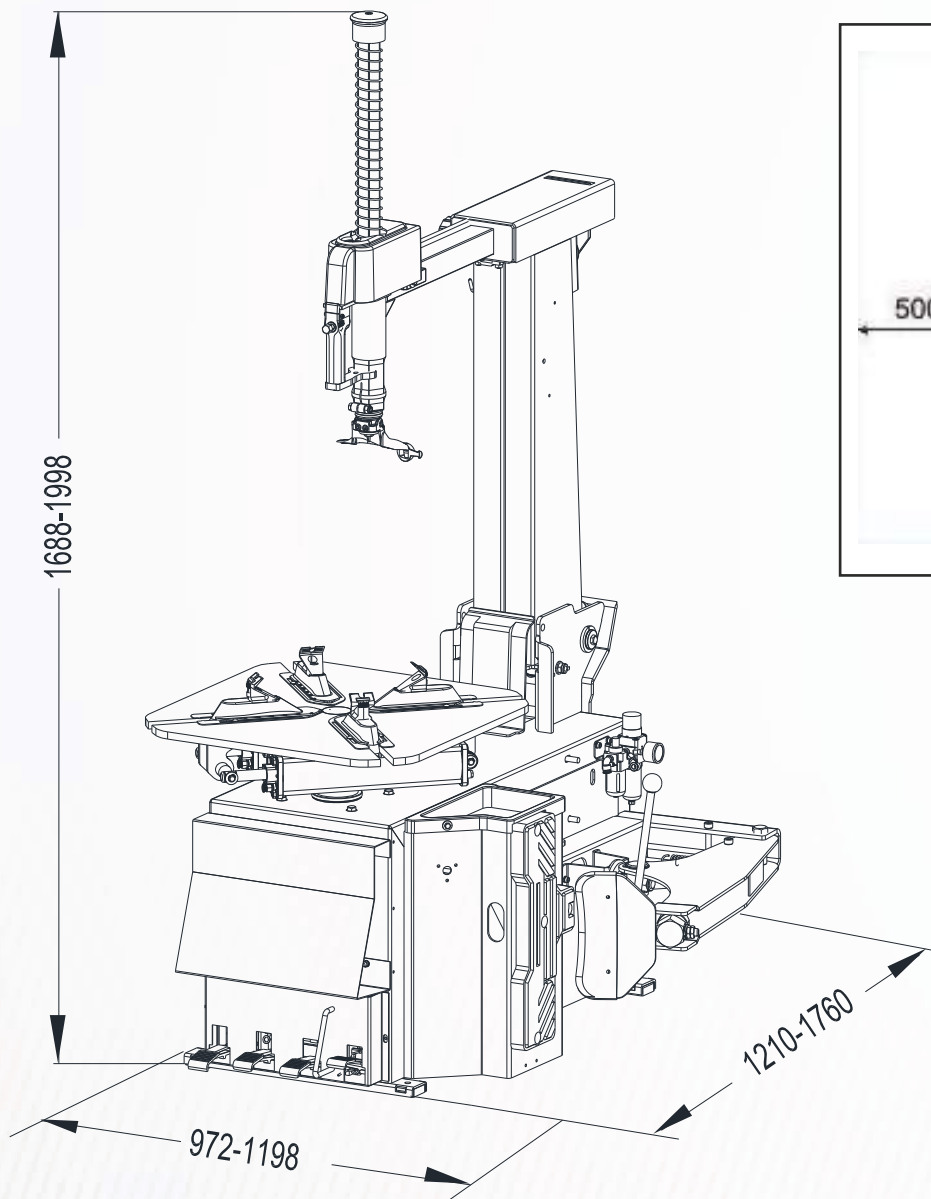
Рисунок 4 Установка стенда
