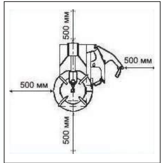
Рисунок 4.1 Установка стенда
