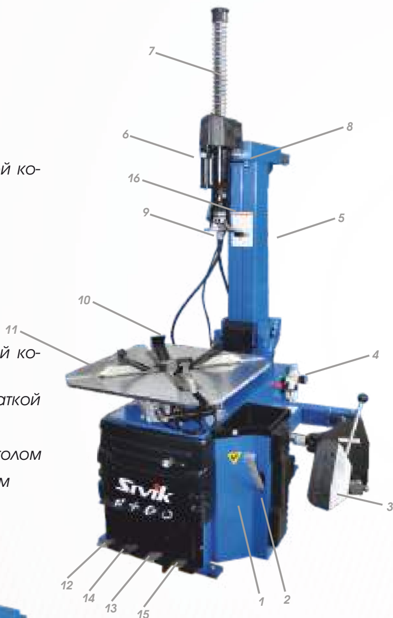
Рисунок 1 Устройство станда
