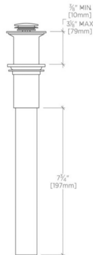
SIDE VIEW SCALE: 3"=1'-0"
