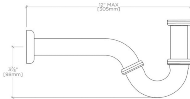
SIDE VIEW SCALE: 3"=1'-0"
