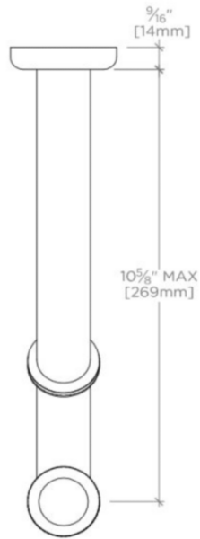
TOP VIEW SCALE: 3"=1'-0"
