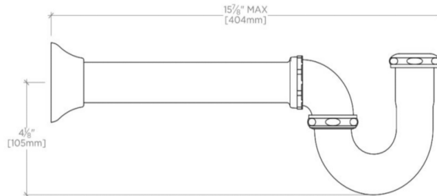
SIDE VIEW SCALE: 3"=1'-0"
