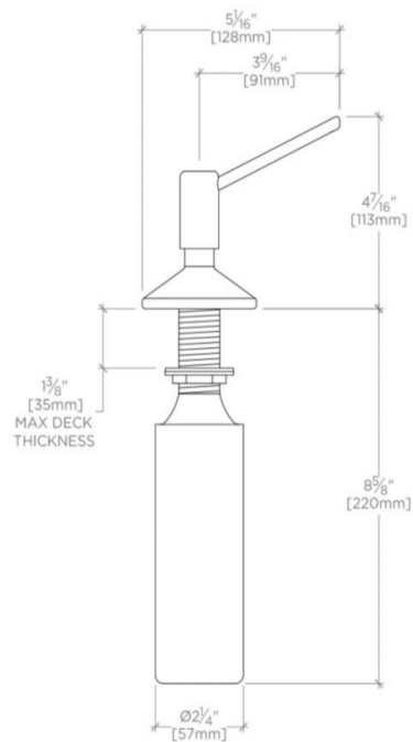
SIDE VIEW SCALE: 3"=1'-0"
