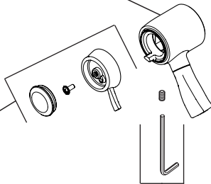
RP52585 ▲ Temperature Knob, Cover & Screw Perilla de la Temperatura, Cubierta y Tornillo Poignée de Réglage de Température, et Vis
