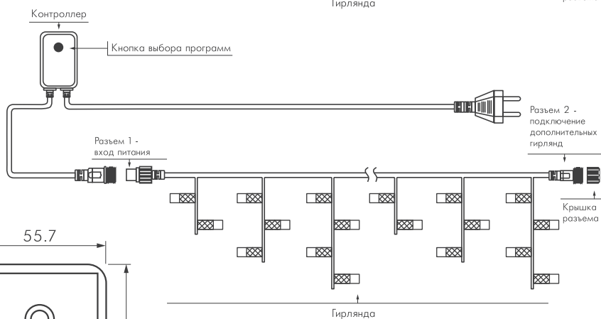
Рис. 1. Схема подключения контроллера.
