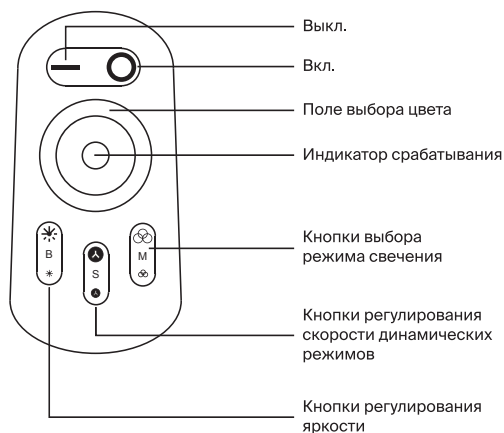
Рис. 2 назначение кнопок пульта управления
