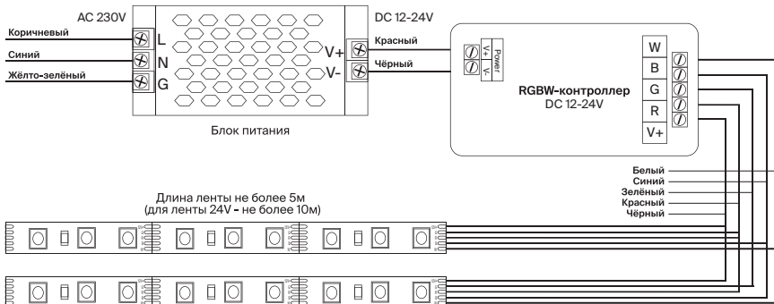
Рис. 1 схема подключения контроллера
