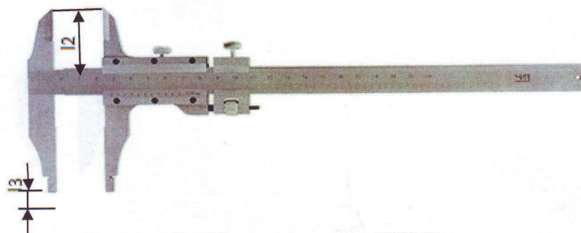
Рисунок 2 – Штангенциркуль ШЦ-II
