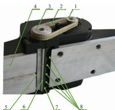
1-ведущий шкив; 2-ремень; 3-ведомый шкив; 4-передняя опорная подошва; 5-фреза; 6-нож; 7-прижимная пластина; 8-прижимные болты
