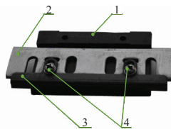
1-приспособление; 2-нож; 3-ограничительная скоба; 4-винты
