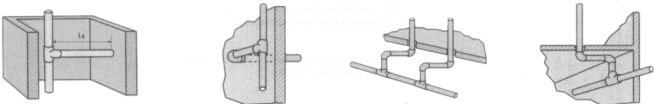
рис. 11: Примеры различных способов компенсации линейного расширения пластикового трубопровода на практике.
