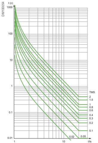
Кривая чрезвычайно обратно-зависимой выдержки времени МЭК (МЭК/ET или МЭК/C)
