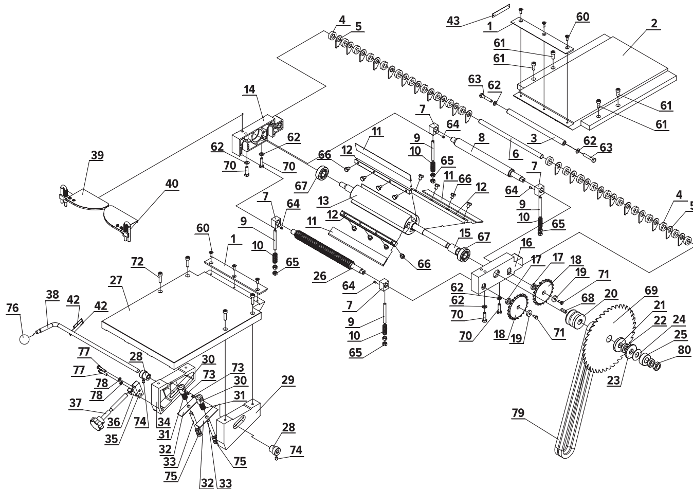
Схема сборки № 4
