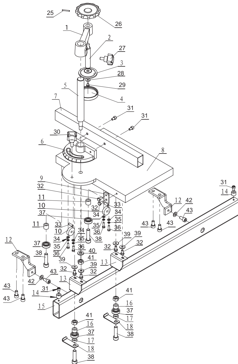
Схема сборки № 1
