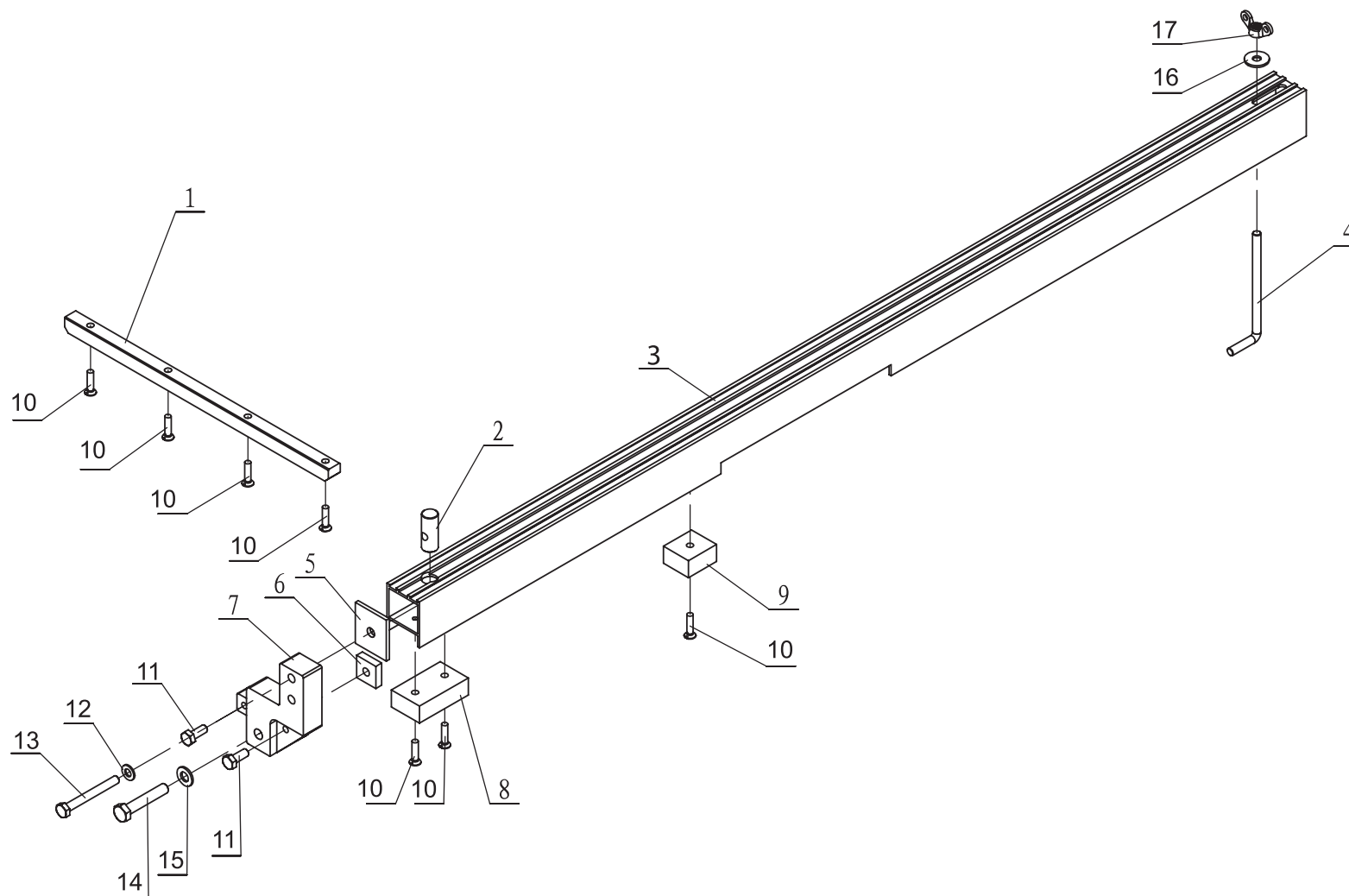
Схема сборки № 3
