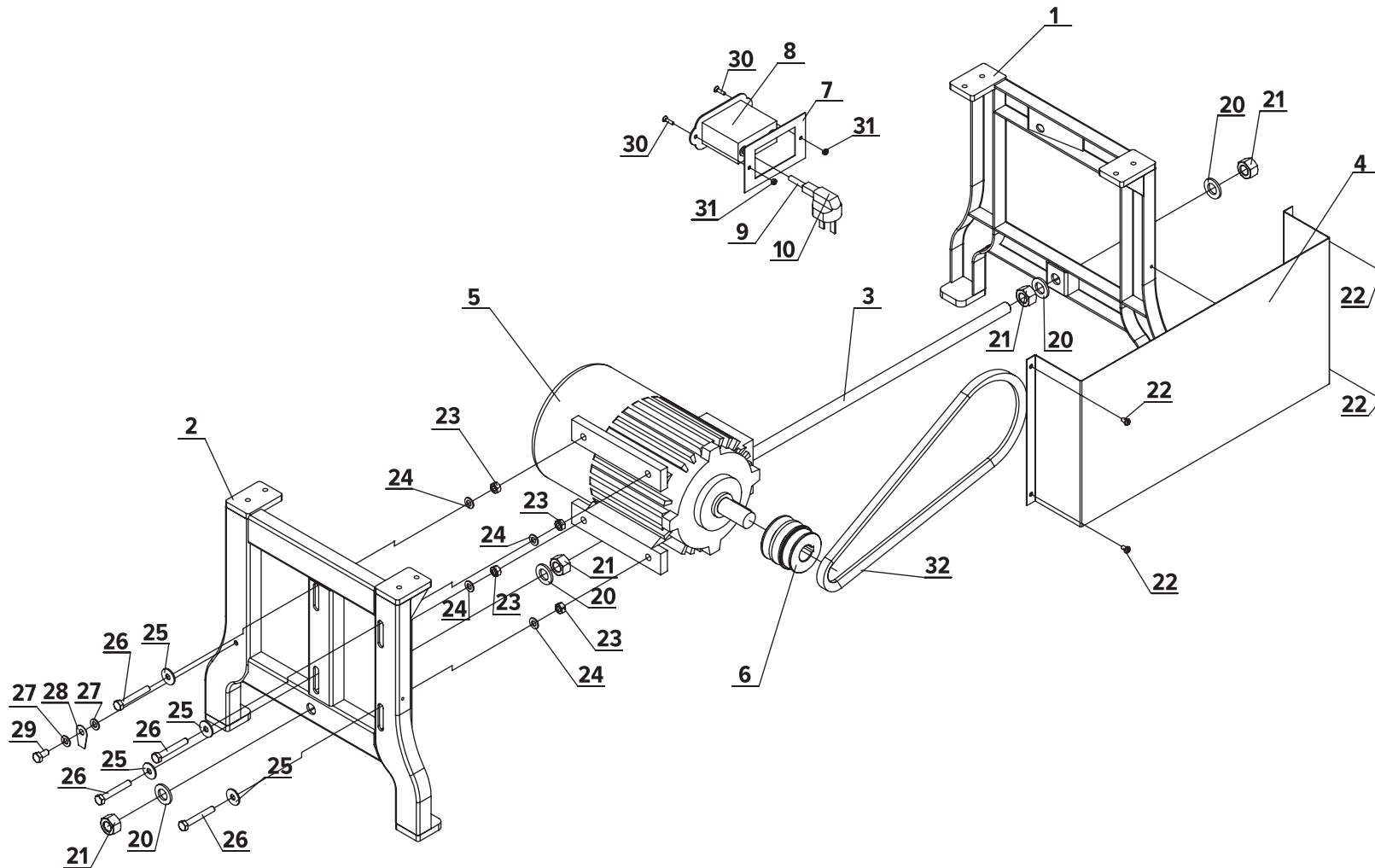
Схема сборки № 5
