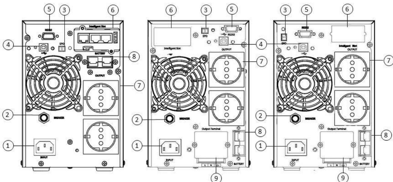
Рис.3 Задняя панель ИБП серии ONLINE PLUS 1000/2000/3000.
