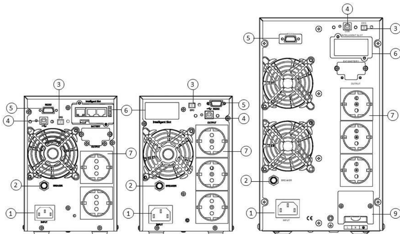
Рис.2 Задняя панель ИБП серии ONLINE 1000/2000/3000.
