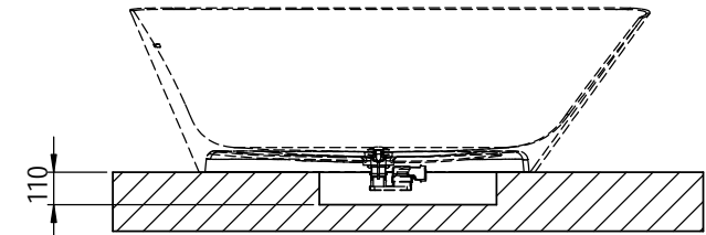
DIMENSIONI FORO POZZETTO FLOOR RECESS SIZE
