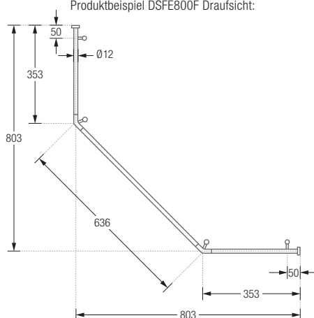
Produktbeispiel DSFE800F Draufsicht:
