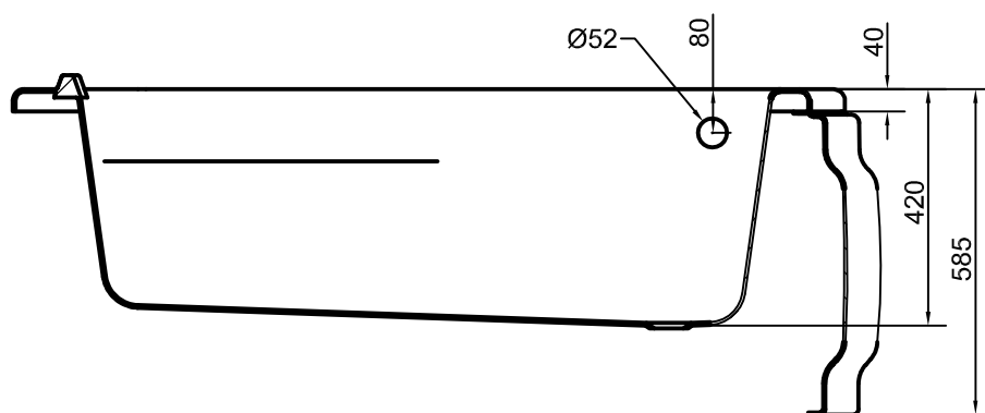
A-A ( 1 : 10 )
