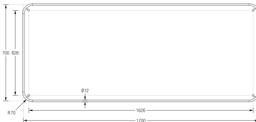
Produktbeispiel DSRE1700-700 Draufsicht:
