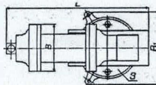
1 - губка подвижная; 2 - корпус; 3 - плита поворотная; 4 - рукоятка
