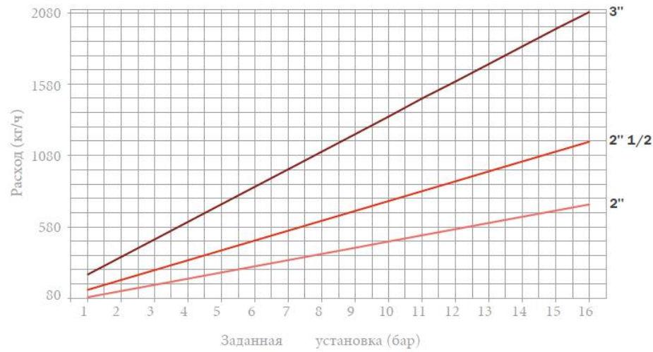
Графики производительности по насыщенному пару
