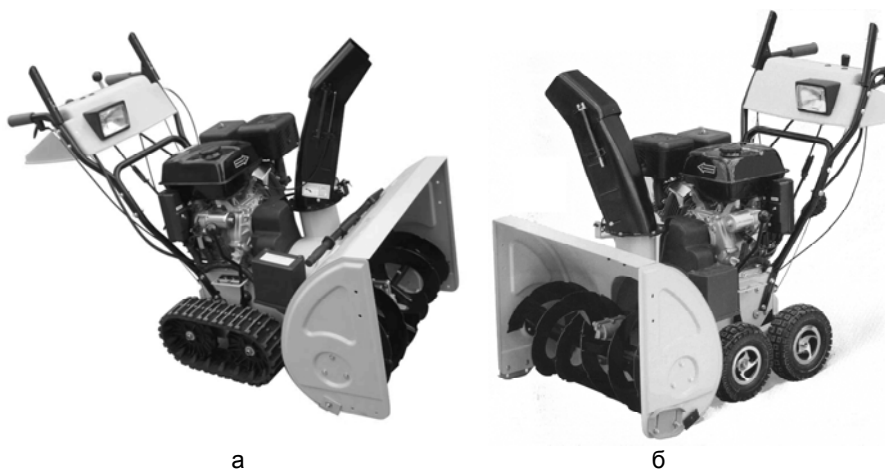
Рис. 1. Механизированные снегоуборщики с двигателем внутреннего сгорания а-МST901Q; б- MST1101Q.
