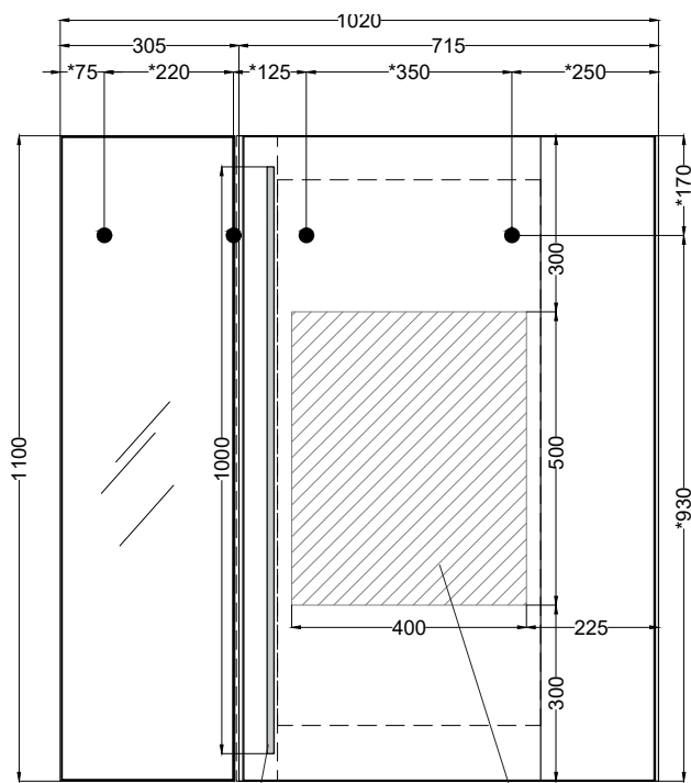
Area nella quale è possibile collocare l'impianto elettrico \ Area where you can locate the electrical system
