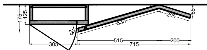
Area nella quale è possibile collocare l'impianto elettrico \ Area where you can locate the electrical system
