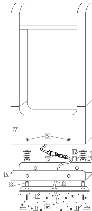
Рис. 1. Установка и подключение светильника.
