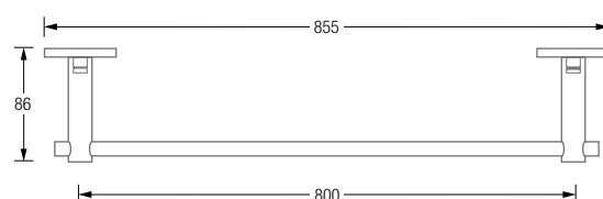
Produktbeispiel HS20-80-800-K55 Draufsicht:
