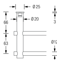
Produktbeispiel HS20-140D800 Detailansicht:
