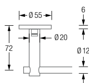
Produktbeispiel HS20-80-800-K55 Detailansicht:
