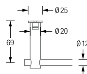
Produktbeispiel HS20-80-800 Detailansicht:
