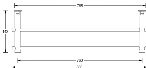
Produktbeispiel HS20-140D800 Draufsicht:
