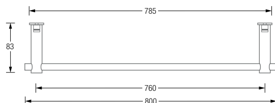
Produktbeispiel HS20-80-800 Draufsicht:
