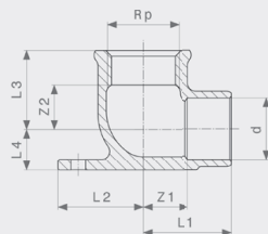
Водорозетка - бронза Модель 94471G
