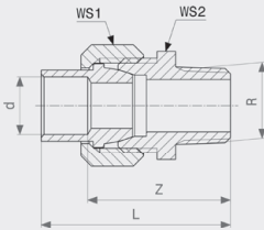
Соединительный элемент резьбовой разъемный - бронза Модель 94343G
