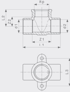
Тройник-водорозетка - бронза Модель 94490G
