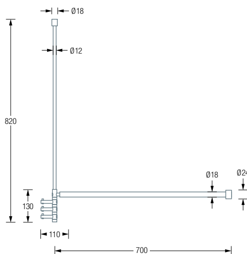
T3L Seitenansicht:
