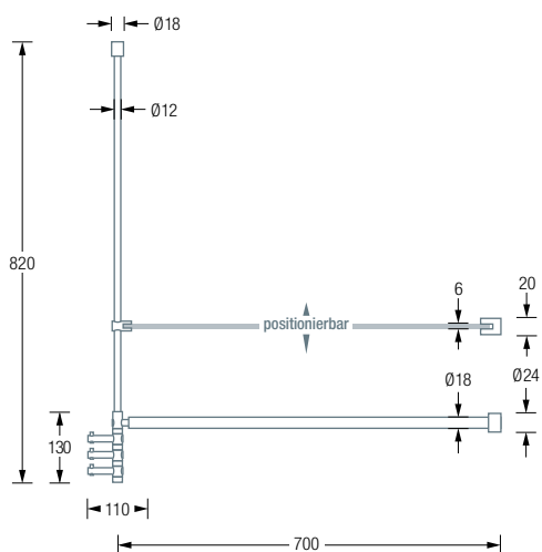
T3LG Seitenansicht:
