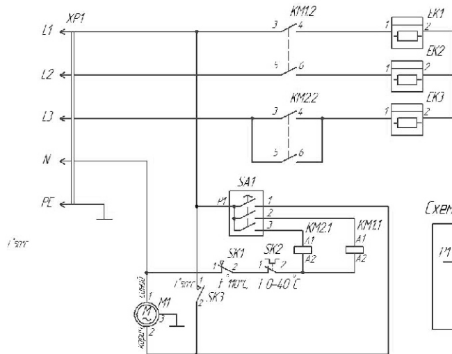
Рис. 1 Схема электрическая
