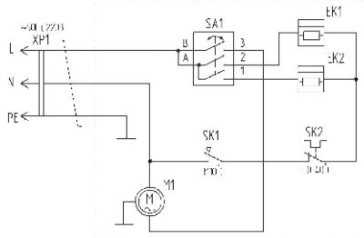
Схема электрическая QS 3; QSE 3020
