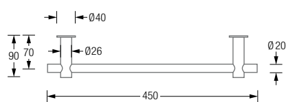
WG26-450 Draufsicht:
