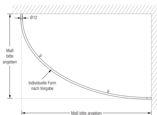
DSGE12 Draufsicht:
