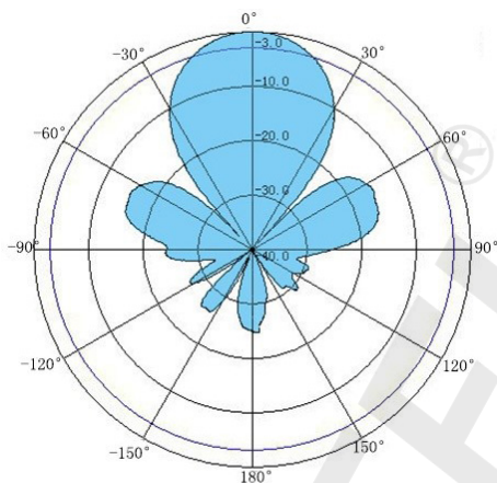
ГОРИЗОНТАЛЬНАЯ ПЛОСКОСТЬ
