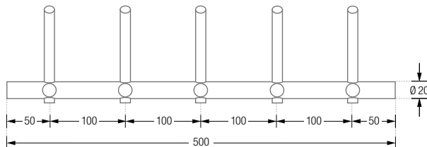
HLS5H-B Frontansicht:
