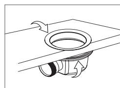
joint autofix double : maintient la bonde sur le receveur et garantit l'étanchéité
