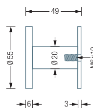
HA3-R55S55-B Seitenansicht:
