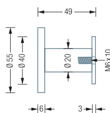
Verklebung:
