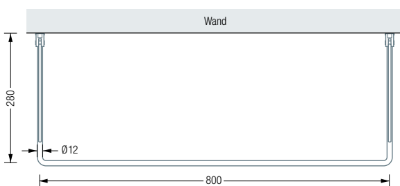
GU1-800 Draufsicht:
