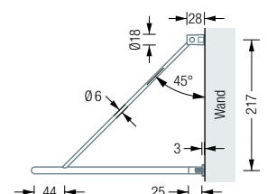
GU1-1600 Seitenansicht:
