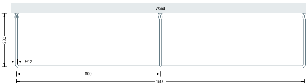
GU1-1600 Draufsicht:
