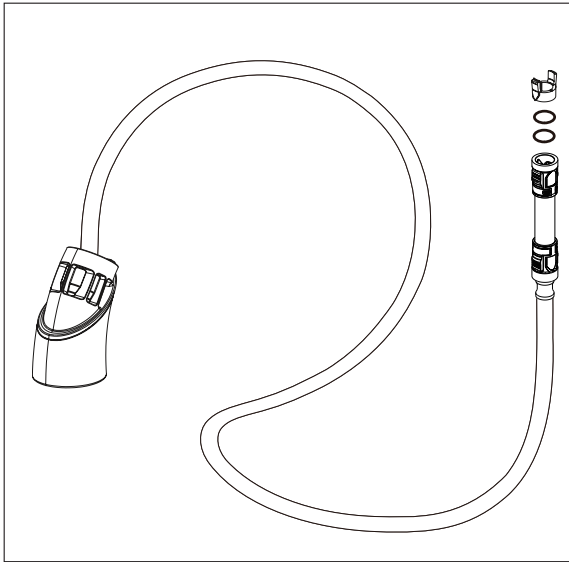
RP100234▲ Hose Assembly, Wand, Clip & O-Rings Montaje de la manguera, varita, clip & O-rings Ensemble de tuyaux, baguettes, clips et joints toriques
