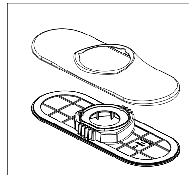
RP101309▲ Escutcheon & Gasket (3 Hole) Chapetón y Empaque (3 agujeros) Boîtier et Joint (3 trous)
