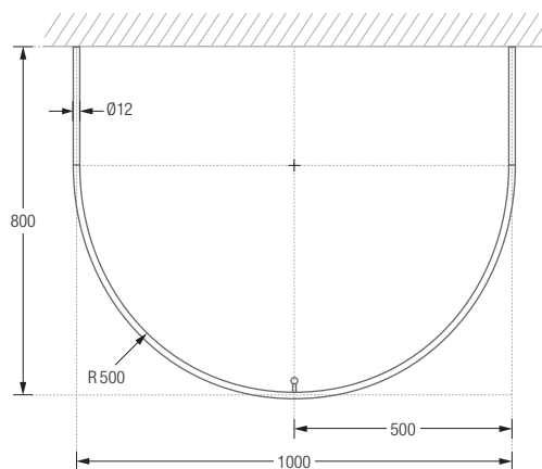
Produktbeispiel DR500HD800 Draufsicht:
