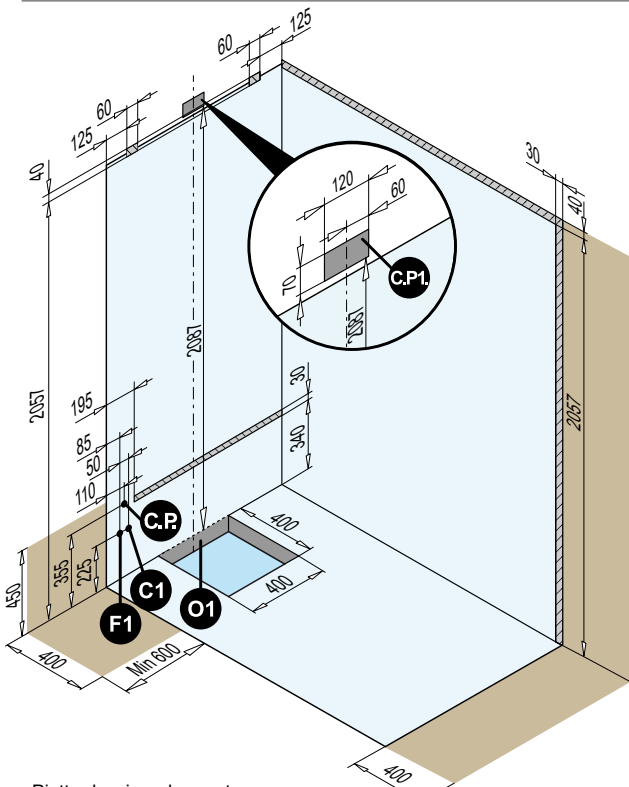
Piatto doccia - shower tray Duschtaße - Platos de ducha - Receveurs de douche
