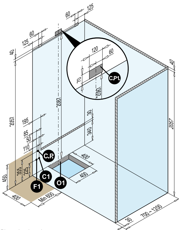
Piatto doccia - shower tray Duschtaße - Platos de ducha - Receveurs de douche
