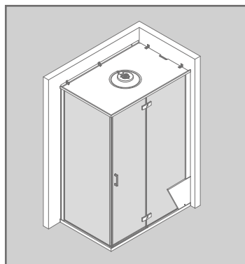
AD ANGOLO_CORNER ECKE_ANGULAR_EN ANGLE
