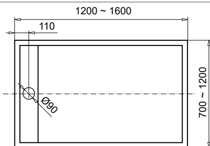
Piatto doccia - shower tray Duschtaße - Platos de ducha - Receveurs de douche
