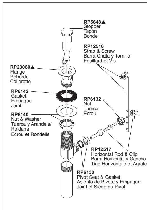
RP26533▲ Metal Pop-Up Assembly Less Lift Rod Ensemble de Metal del Desagüe Automático Menos la Barra de Alzar Renvoi Mécanique en Métal Sans la Tige de Manoeuvre
