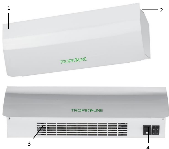
Рис.1. Устройство прибора
